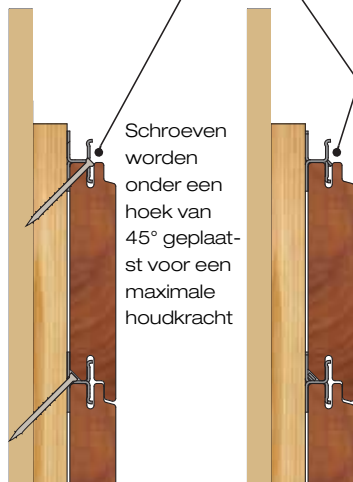
SECTIE A-A
