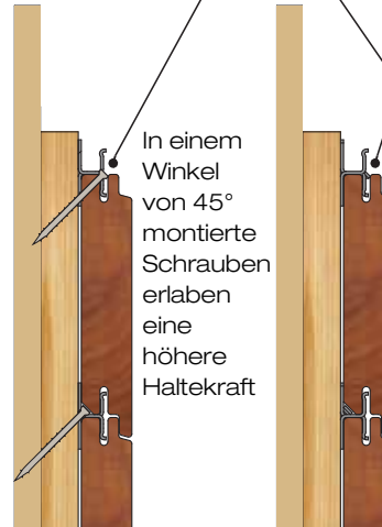
ABSCHNITT A-A
